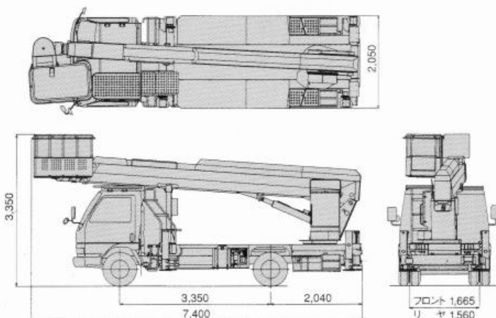
外形寸法図(単位%)
